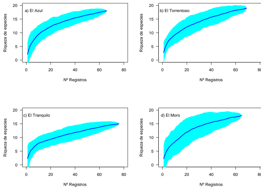
Figura 7: Curvas de rarefacción de especies de aves a partir de los equipos acústicos. Se presenta el ajuste de la curva con el intervalo de confianza del 95%. En a) EL Azul, b) El Torrentoso, c) EL Tranquilo y d) El Moro
